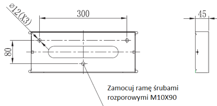
Rama montażowa modeli Growatt 4000UE-6000UE
