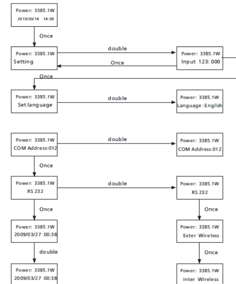
Schemat poruszania się po menu ustawień parametrów
