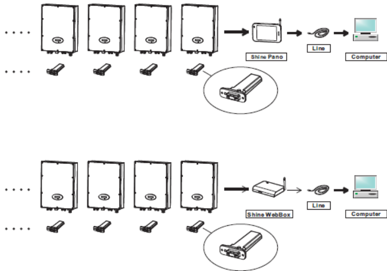
Połączenie interfejsu RS232 z bezprzewodowym rejestratorem danych i internetem.
