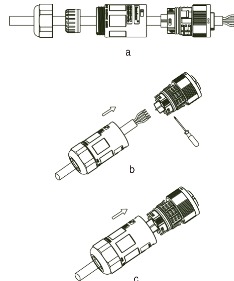
Rys. 6.2 Schemat połączeń wyjścia AC
