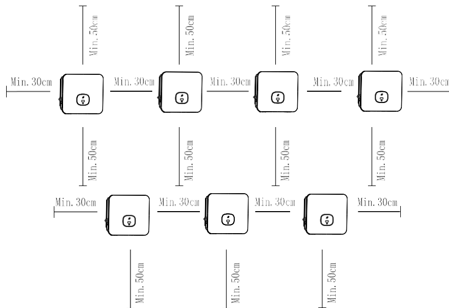
Rys. 5.3 Wymiary montażowe dla wielu falowników
