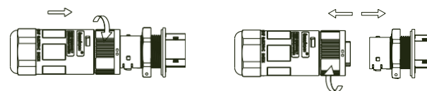
Rys. 6.3 Schemat podłączenia zacisku AC
