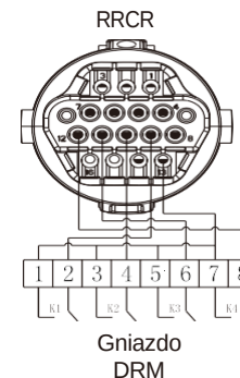
Rys. 6.20 Połączenie falownik - RRCR
