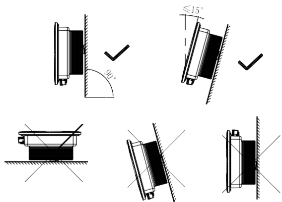
Rys. 5.1 Schemat montażowy
