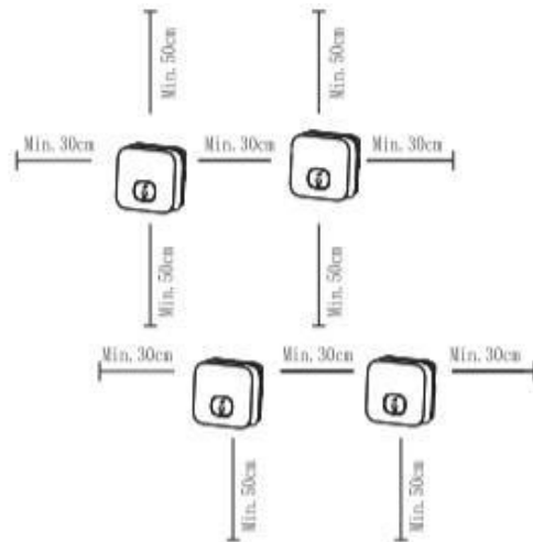
Minimalne odległości dla falowników szeregowych
